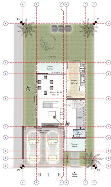
VUE EN PLAN RDC
